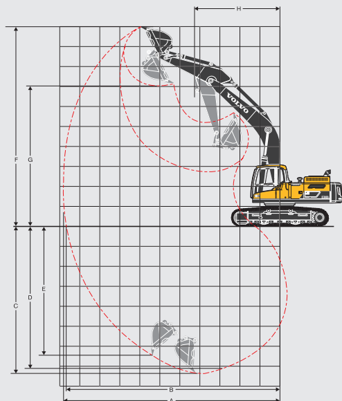
Maschine mit Mono-Ausleger
