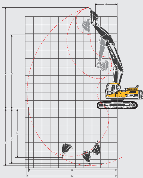
Maschine mit Verstellausleger (2-teilig)
