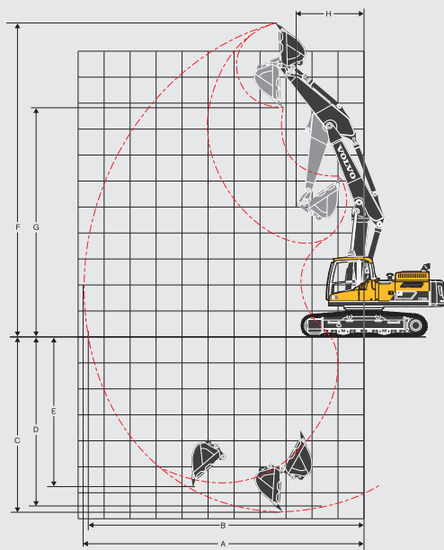
Machine avec flèche articulée
