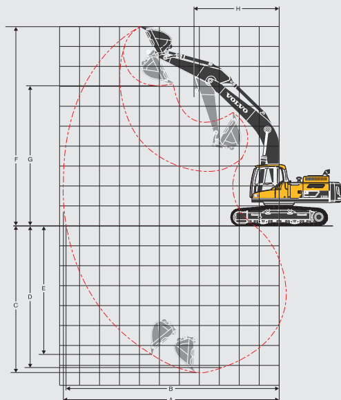
Machine avec flèche monobloc
