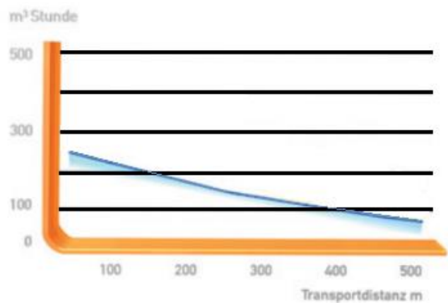
Leistungsdiagramm
