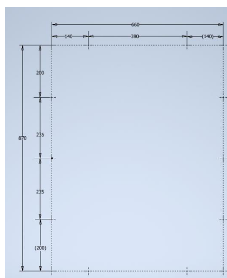
MSP1500R_2000R (660x870)
