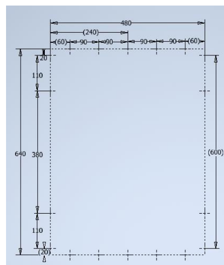
VRG50 (480x600/640)
