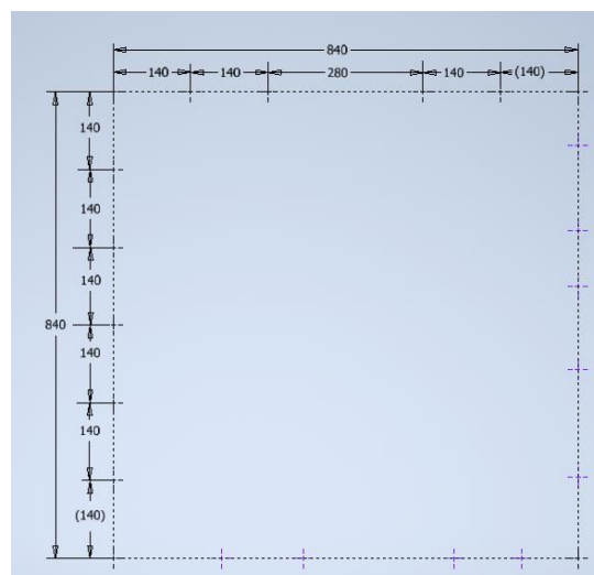
HCS65 (840x840)
