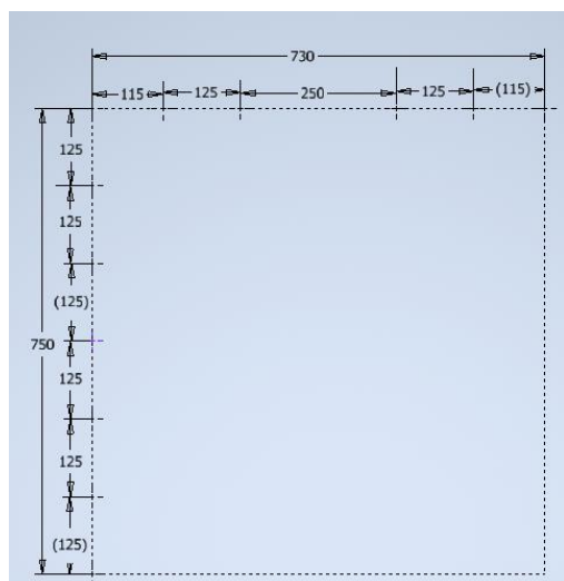
HCC50 (730x750)
